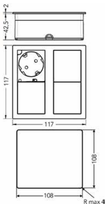
Inbouwstopcontacten Versahit
